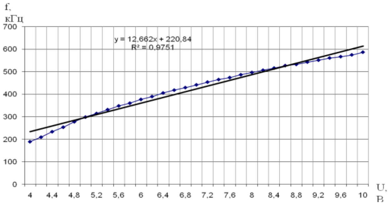
Рисунок 2 – Залежність частоти вихідних імпульсів генератора від керуючої напруги
