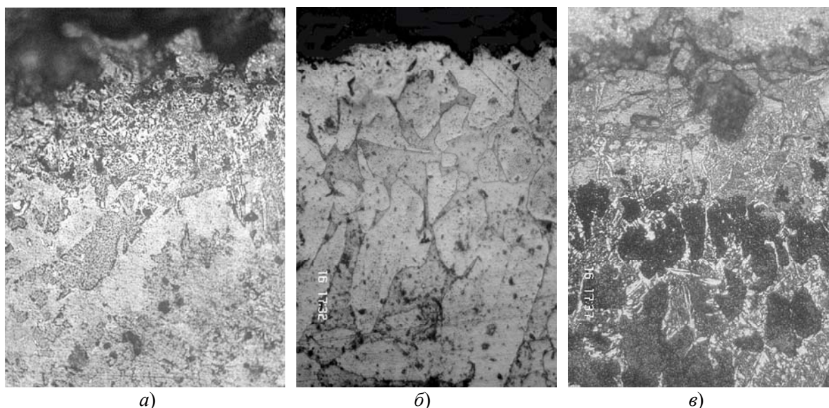
Рисунок 1 – Микроструктуры многокомпонентных покрытий, полученных методом СВС на сплавах меди, \times 100
